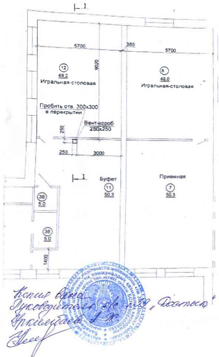
Фрагмент плана 2-го этажа, с вентиляционной системой из кухни
