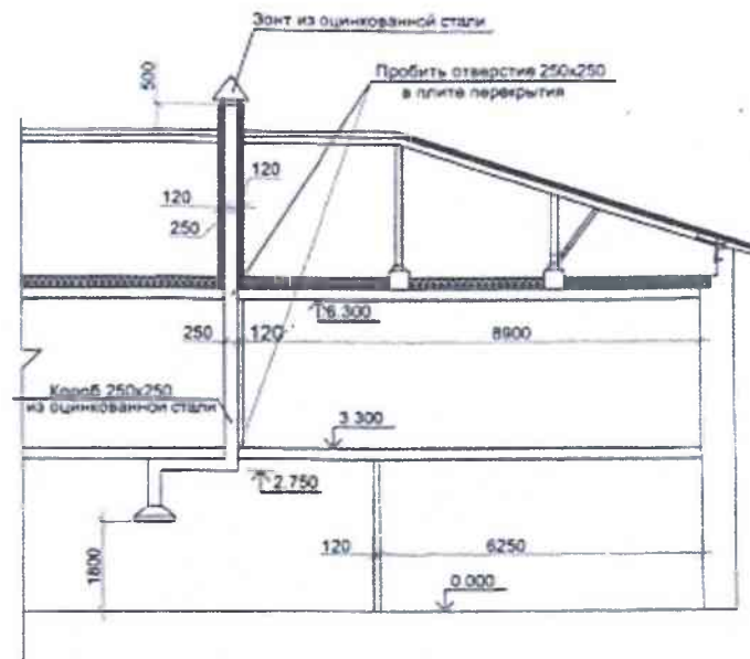
Разрез 1 - 1
